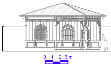
Elevação 01
