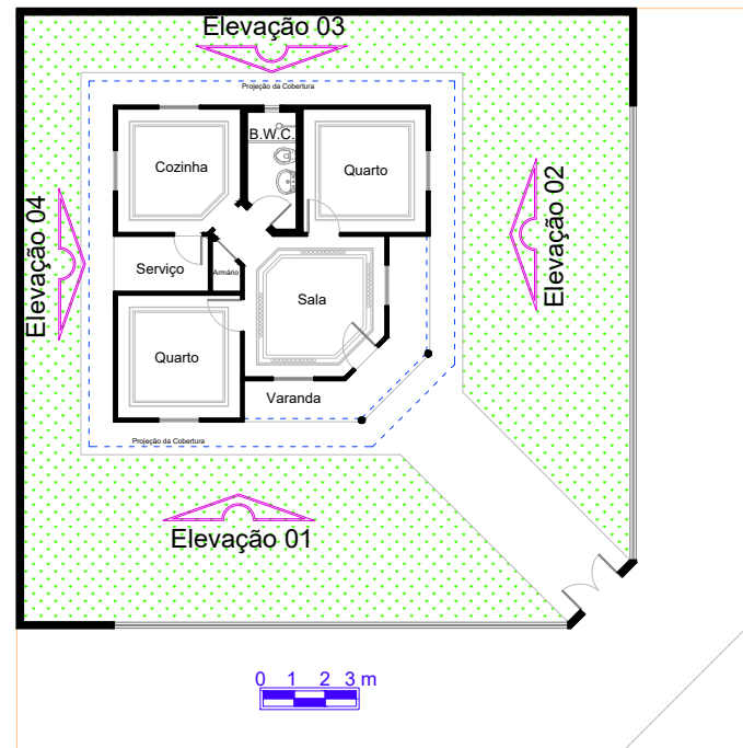
Planta
