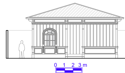
Elevação 04
